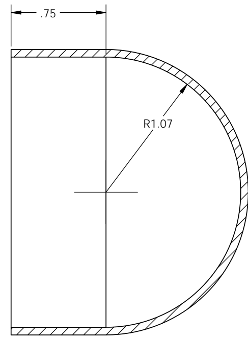
SECTION A-A SCALE 2 : 1
