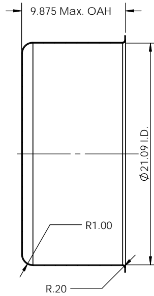
SECTION A-A SCALE 1 : 6
